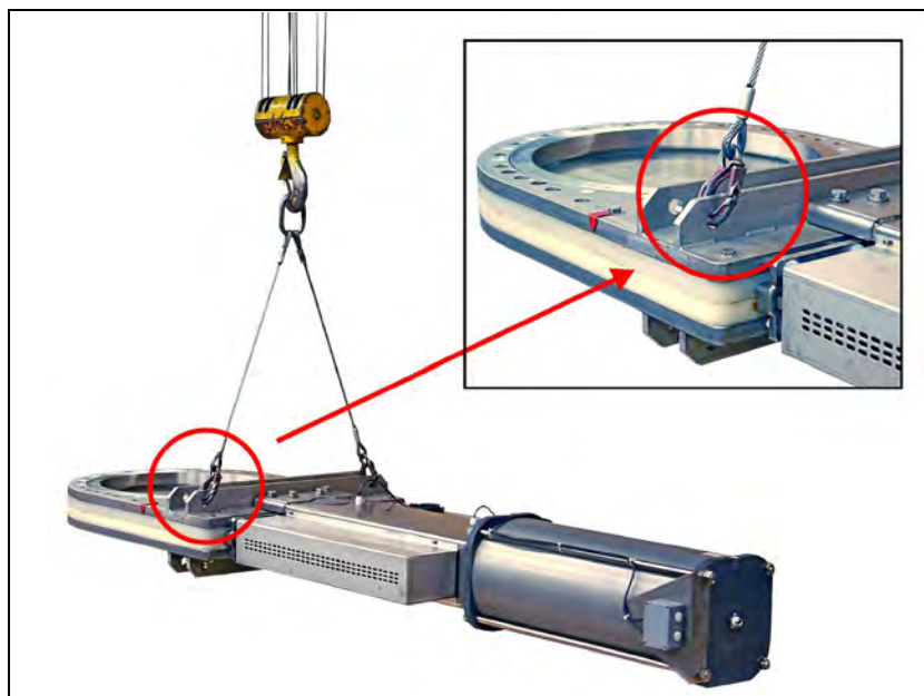
Punkt zamocowania na obudowie
